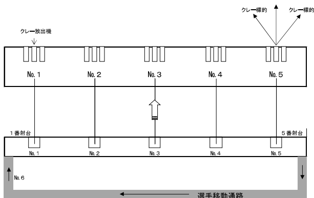
トラップ射撃場構造図
