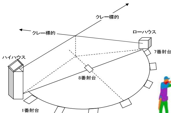
スキート射撃場立面構造図
